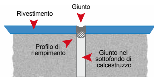
Giunto di contrazione o di costruzione
