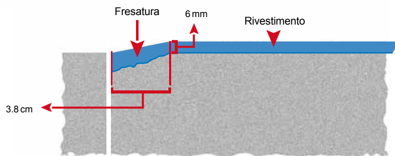
Punto di delimitazione di un pavimento in resina
