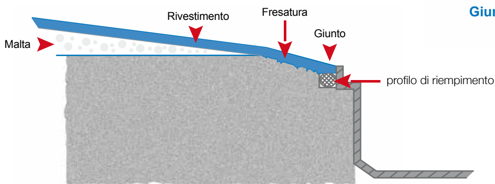
Canalina prefabbricata
