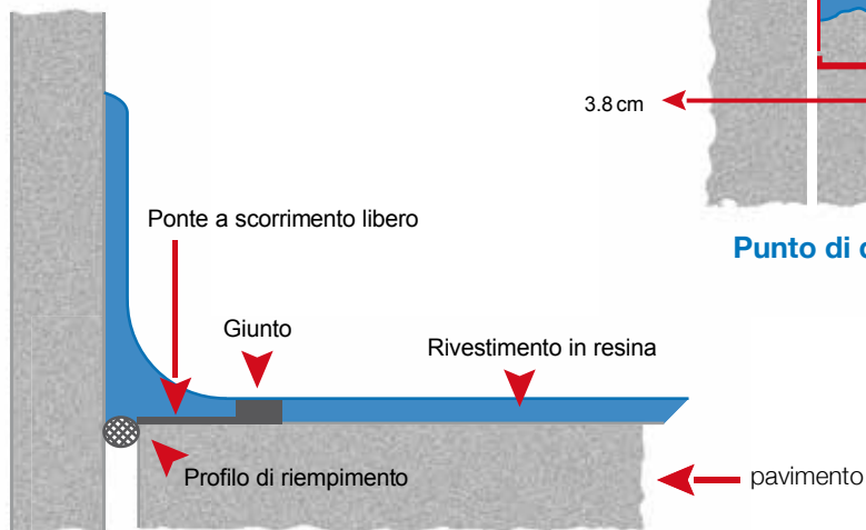
Guscia standard pavimento / parete esterna
